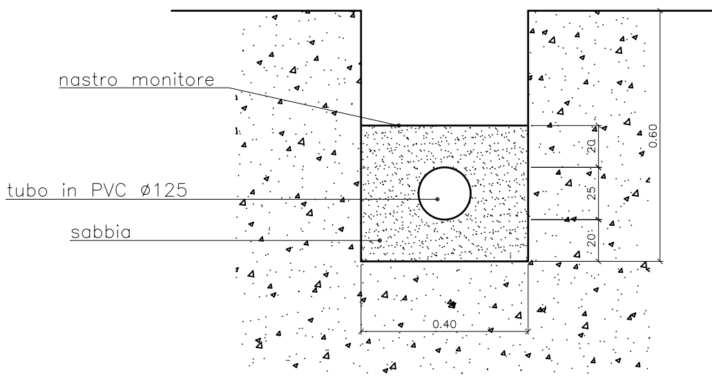
SEZIONE CONVENZIONALE DI SCAVO PER TUBAZIONI TELECOM SU MARCIAPIEDE
