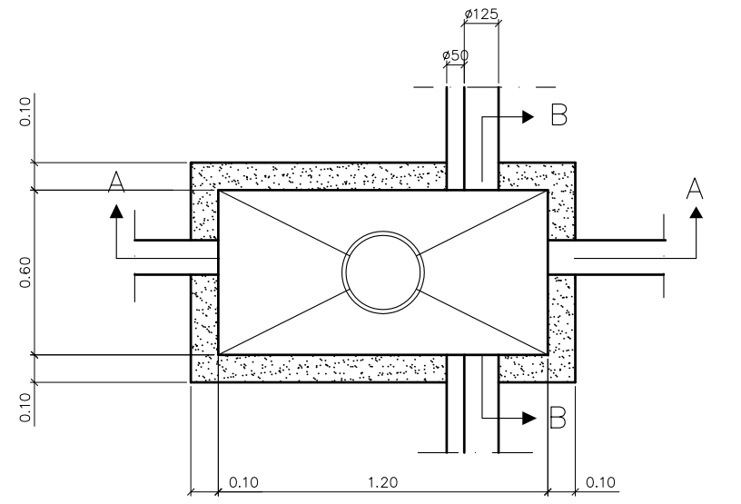
POZZETTO DOPPIO TELECOM SU MARCIAPIEDE
