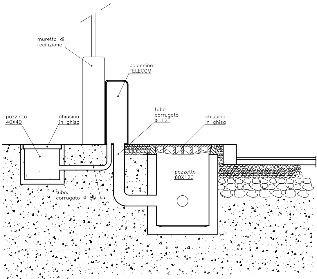
PARTICOLARE POZZETTO E COLONNINA TELECOM SU MARCIAPIEDE
