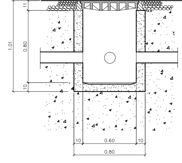
SEZIONE B-B
