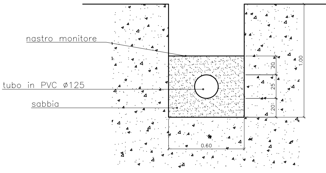
SEZIONE SCAVO TIPO PER TUBAZIONI TELECOM SU STRADA
