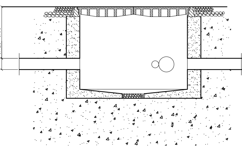
SEZIONE A-A
